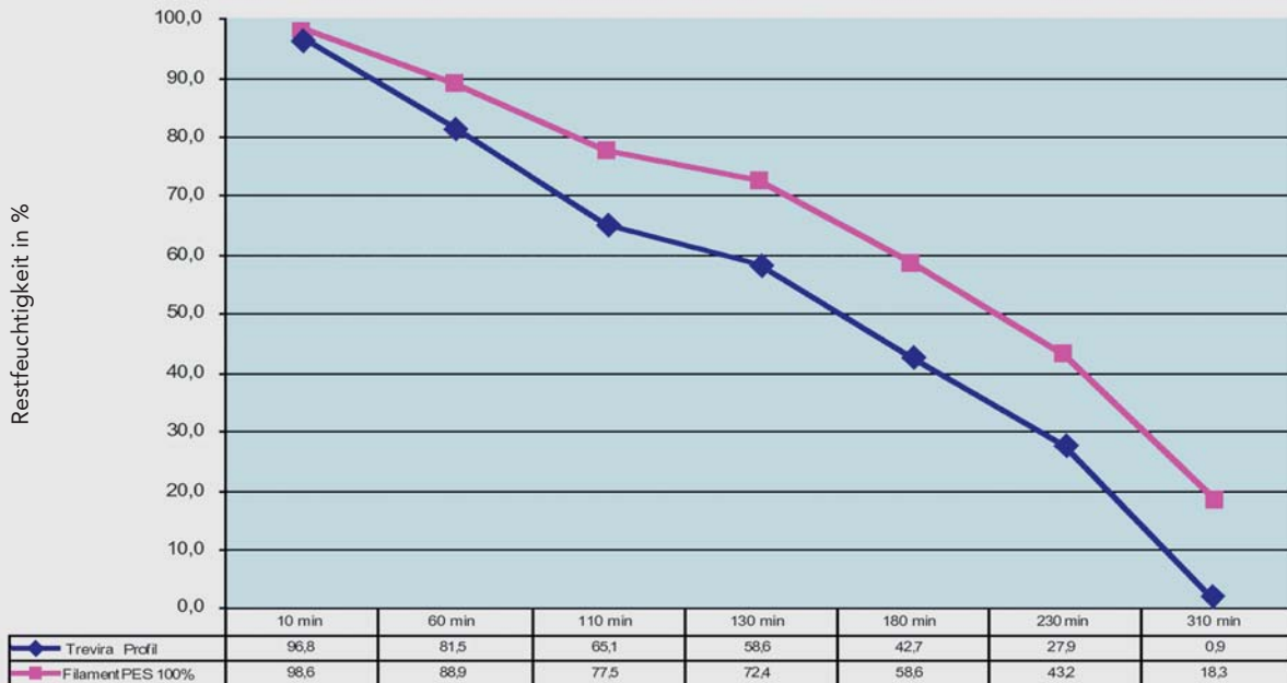
Trocknungszeiten Gewebe – Klimabedingungen: 22°C, relative Luftfeuchtigkeit 56%
